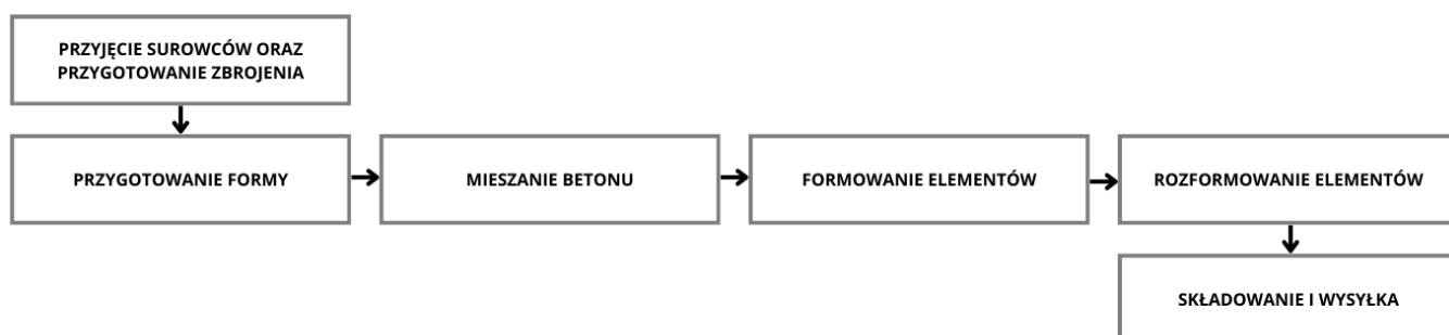
Rysunek 4.1: Uproszczony schemat produkcyjny elementów prętowych zbrojonych
